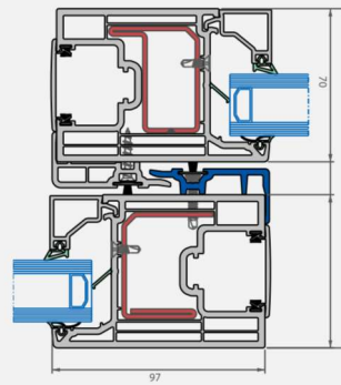
Coupe horizontale
